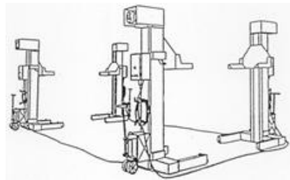
Siirrettävä, pyöristä nostava 4-pilari- nostin, kuormauselimenä nostoha- rukka.
